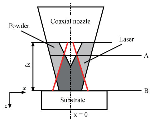
Fig. 2. Powder distribution according to the focal position f_s [19] Рис. 2. Розподіл порошку відповідно до фокусного положення f_s [19]
