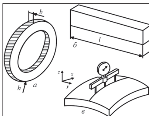
Рис. 9. Методи визначення ЗН: кільця (а); смужок (б); вимірюванням прогину (в)
