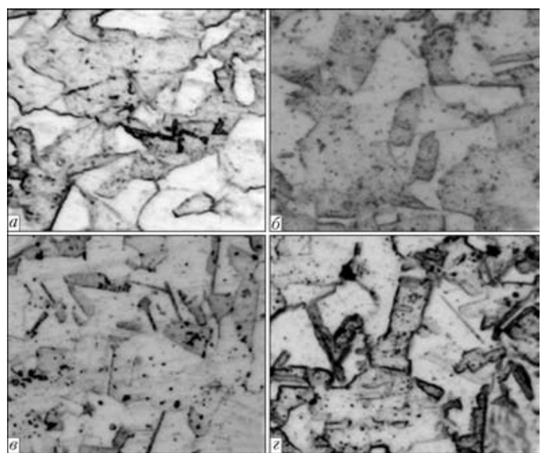
Рис. 3. Микроструктуры (×1000) образца из стали 10X18N10T в зависимости от параметров ИЭТ: а — исходное состояние; б — I=40; в — 80; г — 115 кА
