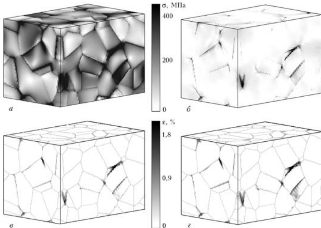
Рис. 9. Интенсивность напряжений ( а, б ) и пластических деформаций ( в, з ) в металле ЗТВ на расстоянии 0,7 мм от линии сплавления ( T^* = 1100\text{ }^\circ\text{C} ) в точках 2 ( а, в ) и 5 ( б, з ) термического цикла (см. рис. 7, в )
