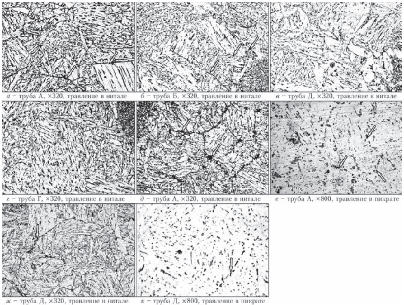
Рис. 1. Микроструктура металла ЗКЗ сварных соединений труб с различным содержанием молибдена и ниобия: a–г — ЗТВ наружного шва; д–к — ЗТВ внутреннего шва, участок повторного нагрева
