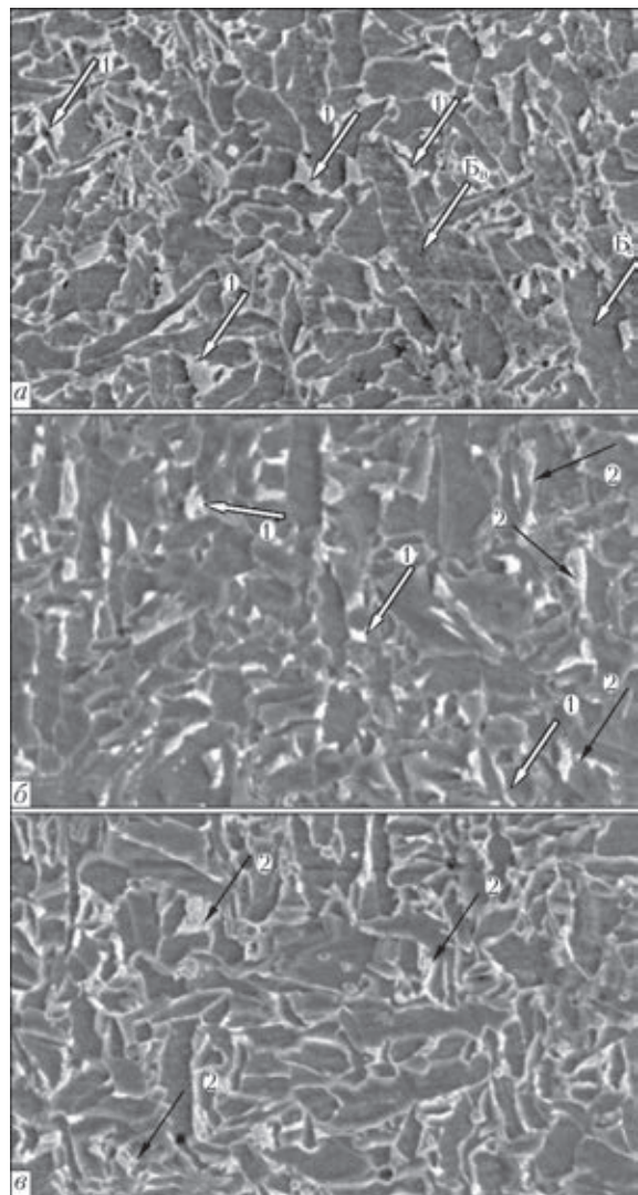
Рис. 5. Морфология и топография МАК-фазы в металле наружных швов с различным содержанием молибдена и ниобия (×3000, растровая микроскопия): а — труба А; б — В; в — Г; 1 — мартенситно-аустенитный комплекс (светлая стрелка); 2 — МАК-фаза (темная стрелка)
