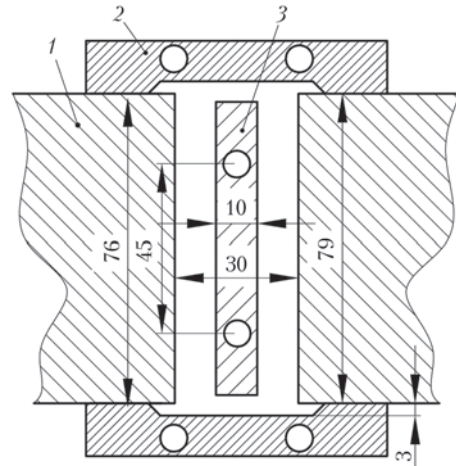
Рис. 2. Геометрические параметры сборки изделий под ЭШС: 1 — свариваемые изделия; 2 — водоохлаждаемая формирующая планка (ползун); 3 — мундштук
