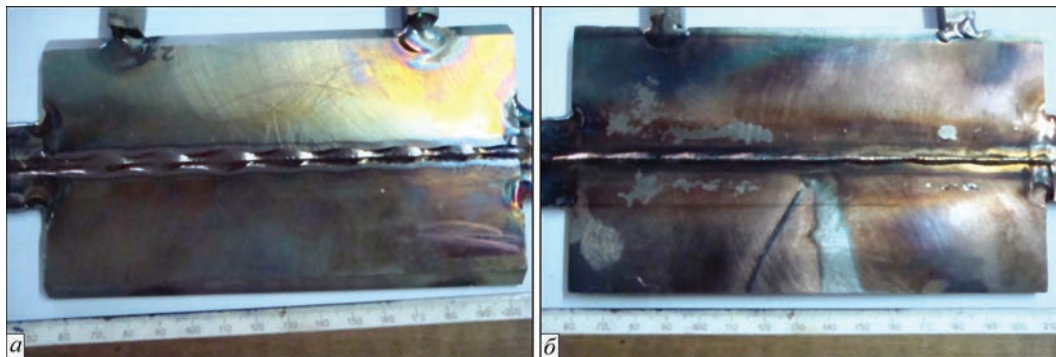
Рис. 1. Общий вид сварного соединения сложнолегированного высокопрочного титанового сплава, полученного ЭЛС: а — лицевая, б — корневая сторона
