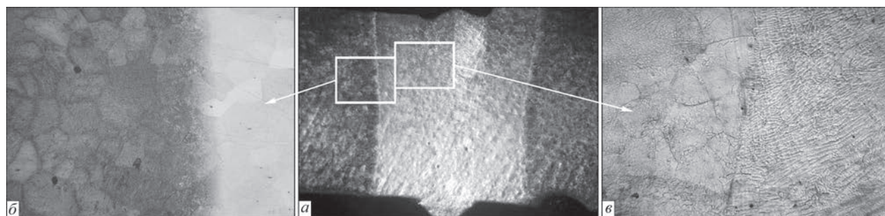
Рис. 3. Структура сварного соединения образца № 1: а — общий вид ( \times 10 ); б — микроструктура ОМ ( \times 50 ); в — микроструктура шва и ЗТВ ( \times 100 )
