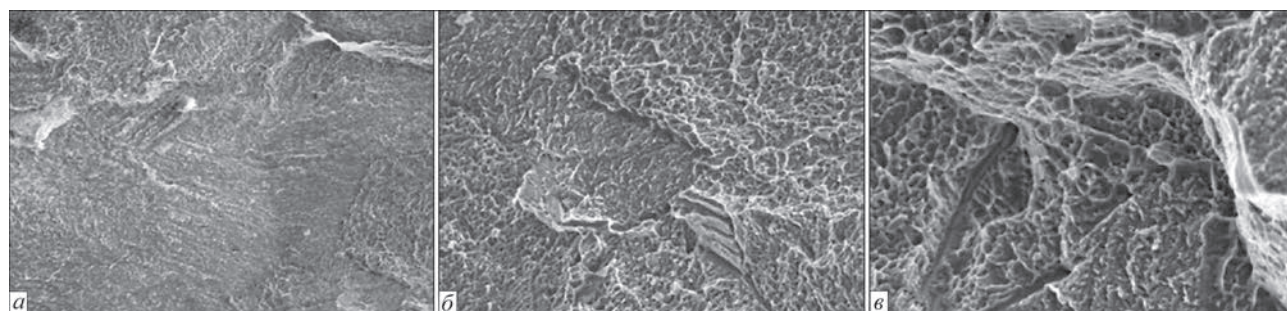
Рис. 4. Фрагменты поверхности разрушения образца № 1: а — межзеренное ( \times 300 ); б — внутриверенное в сочетании с отрывом ( \times 500 ); в — ямочного характера с отрывом и вторичными трещинами ( \times 1000 )
