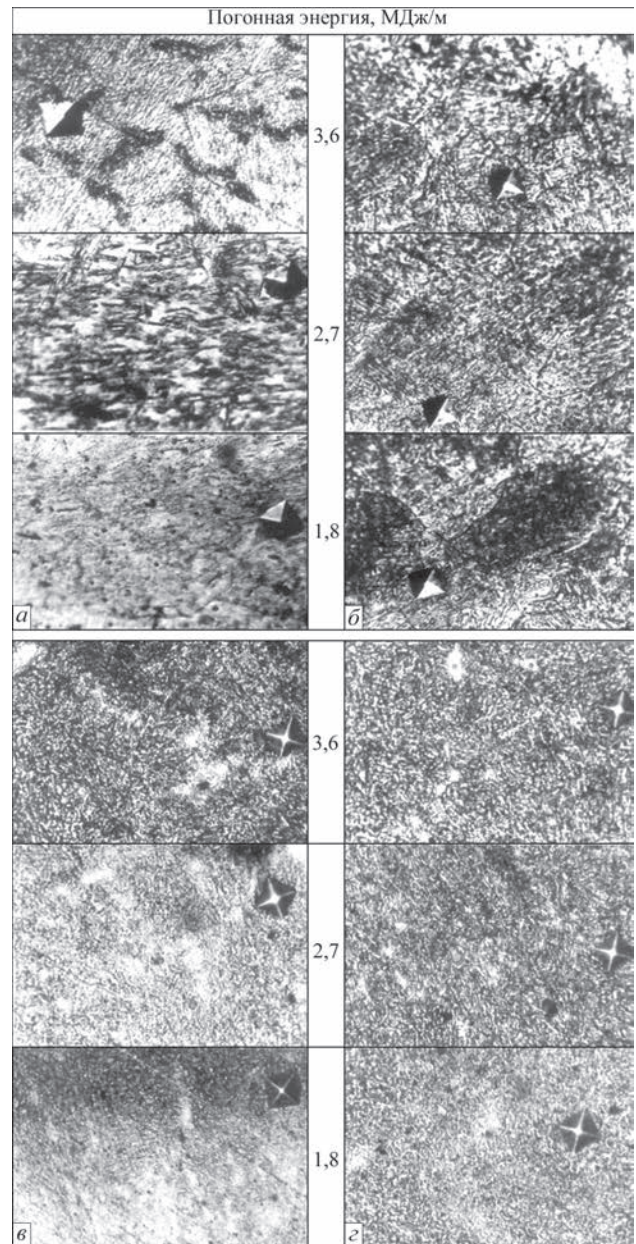
Рис. 6. Микроструктура ( \times 300 ) металла, наплавленного продольной ( a ), перпендикулярной ( б ) лентой, проволочным ( в ) и составным ( г ) электродами с различной погонной энергией
