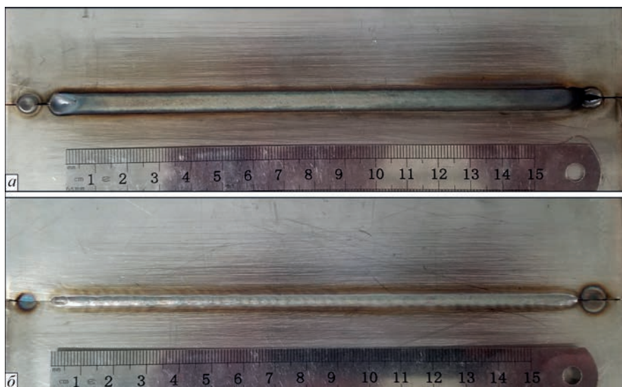
Рис. 3. Внешний вид пластин стали SUS304 (δ = 3,0 мм), сваренных встык с зазором 0,5 мм между кромками лазерно-микроплазменным способом (мощность излучения P = 1,2 кВт, сварочный ток I = 80 А, напряжение U = 28 В, скорость сварки v = 30 м/ч): лицевая (а) и обратная (б) стороны
