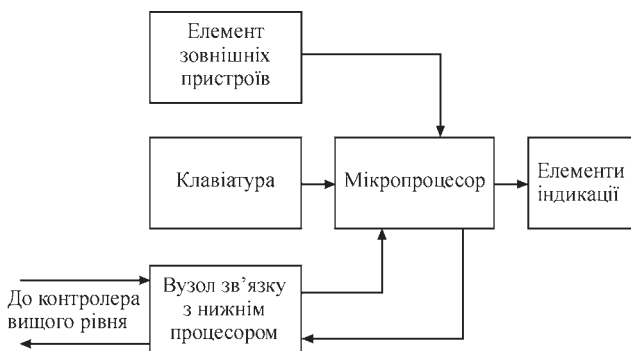
Рис. 8. Структурна схема блоку індикації
