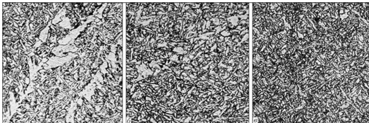
Рис. 13. Микроструктура (×500) металла швов труб из стали класса прочности К60, выполненных с применением различных сварочных материалов: а — Mn-Mo система легирования, кислый плавящийся флюс, полигонального феррита 20...25 %; игольчатого 35...45 %; KV_{-30} = 27...30 Дж/см 2 ; б — Mn-Ni-Mo система легирования, алюминатный агломерированный флюс небольшой основности, полигонального феррита 3...5 %, игольчатого 75...80 %; KV_{-30} = 80...100 Дж/см 2 ; в — Mn-Mo-Ti-V система легирования, алюминатный агломерированный флюс небольшой основности, полигонального феррита менее 1 %, игольчатого 85...90 %; KV_{-30} = 180...200 Дж/см 2
