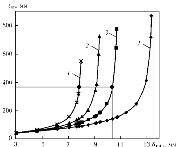
Рис. 17. Зависимость критической длины дефекта типа локального утонения s_{cr} от минимальной допустимой толщины \delta_{min} стенки трубы 1420×20 мм из стали 17Г1С при различном внутреннем давлении: 1 — 4,5; 2 — 5,25; 3 — 6,0; 4 — 7,5 МПа
