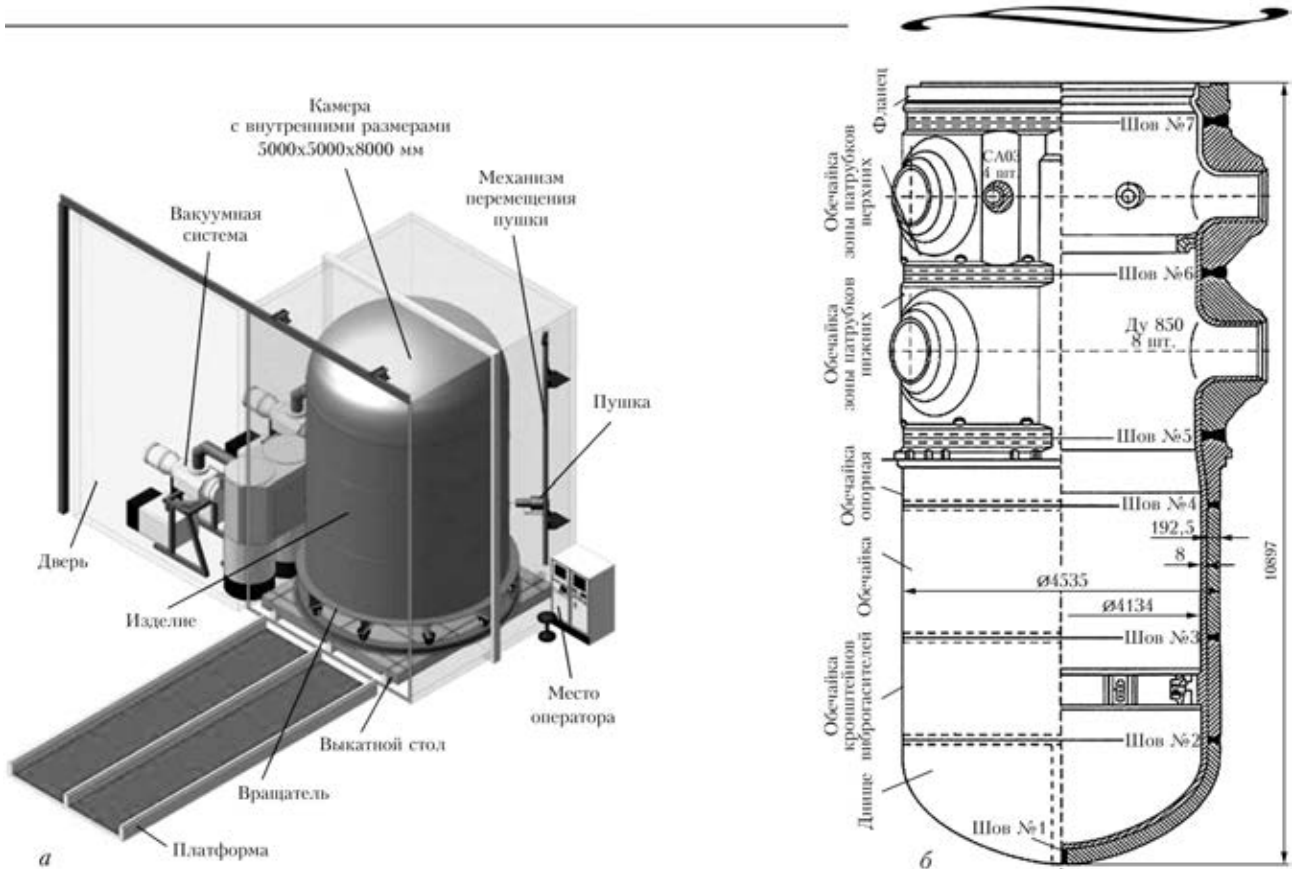
Рис. 7. Принципиальная схема промышленной установки для ЭЛС кольцевых швов корпуса реактора ВВР-1000 (а) и схема корпуса реактора (б)
