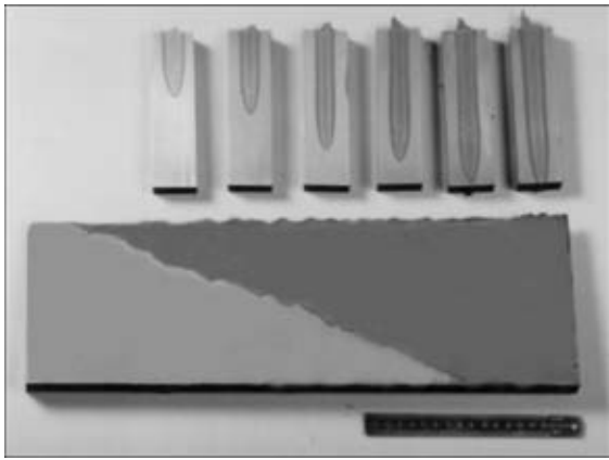
Рис. 5. Макрошлифы участка замыкания кольцевого шва при ЭЛС стали 15X2NMFA толщиной 150 мм
