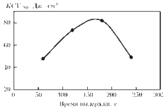
Рис. 15. Зависимость средних значений ударной вязкости от времени выдержки при температуре термической обработки 1000 °С
