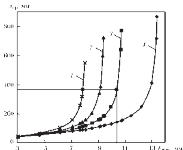
Рис. 17. Зависимость критической длины дефекта типа локального утонения s_{кр} от минимальной допустимой толщины \delta_{мин} стенки трубы 1420×20 мм из стали 17Г1С при различном внутреннем давлении: 1 — 4,5; 2 — 5,25; 3 — 6,0; 4 — 7,5 МПа
