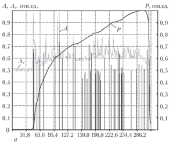
Рис. 19. Одна из точек измерения акустико-эмиссионной активности трубопровода промежуточного перегрева пара Киевской ТЭЦ-6
