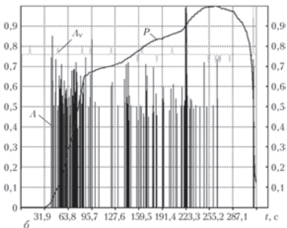
Рис. 18. Сопоставление сигналы акустической эмиссии в растягиваемых образцах из стали 15Х1М1Ф при комнатной температуре (а) и 500 °С (б) (А — амплитуда; A_v — амплитуда непрерывной эмиссии; P — нагрузка)
