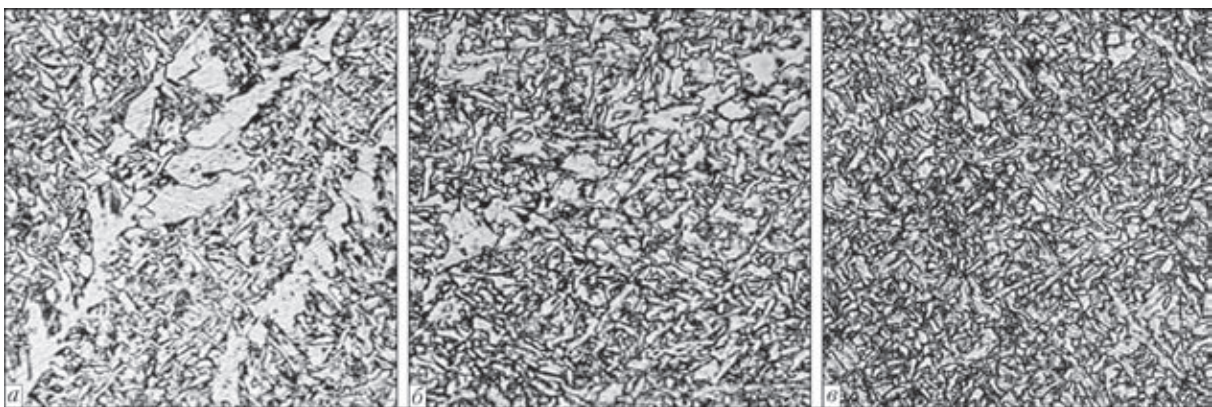
Рис. 13. Микроструктура (×500) металла швов труб из стали класса прочности К60, выполненных с применением различных сварочных материалов: а – Mn–Mo система легирования, кислый плавяный флюс, полигонального феррита 20...25 %; игольчатого 35...45 %; KV_{-30} = 27...30 Дж/см 2 ; б – Mn–Ni–Mo система легирования, алюминатный агломерированный флюс небольшой основности, полигонального феррита 3...5 %, игольчатого 75...80 %; KV_{-30} = 80...100 Дж/см 2 ; в – Mn–Mo–Ti–V система легирования, алюминатный агломерированный флюс небольшой основности, полигонального феррита менее 1 %, игольчатого 85...90 %; KV_{-30} = 180...200 Дж/см 2
