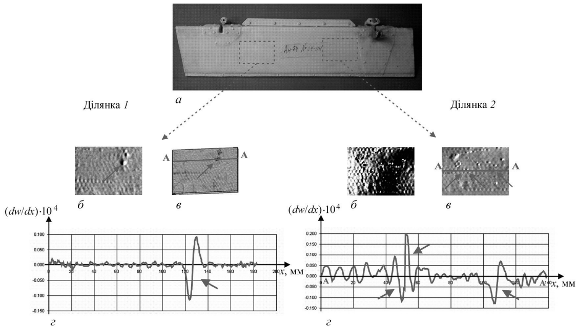
Рис. 4. Ширографічний контроль тримера РВ літака Ан-74 (ділянки 1 і 2) під дією термічного навантаження гарячим повітрям температурою 100 °С впродовж 5 с, величина широзсуву 1 мм уздовж осі OX: а – загальний вигляд елемента; б – широграма контрольованої ділянки; в – поверхня розподілу похідної dw/dx на досліджуваній ділянці з нанесеним досліджуваним перерізом; г – крива зміни похідної dw/dx уздовж обраного перерізу на ділянці з дефектом А-А (місця дефектів позначені стрілками)
